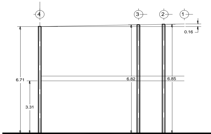
ALZADO LATERAL
